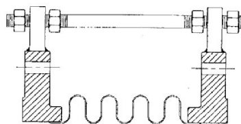
Detalle de Tirante limitador / Limit Rods detail
